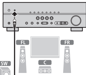
YPAO-Mikrofon Hörposition
