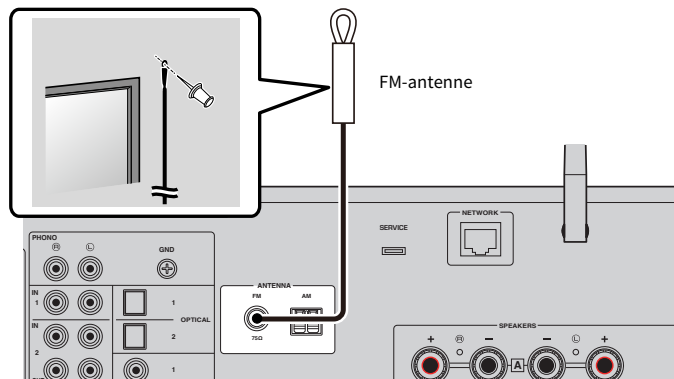
Achterpaneel
