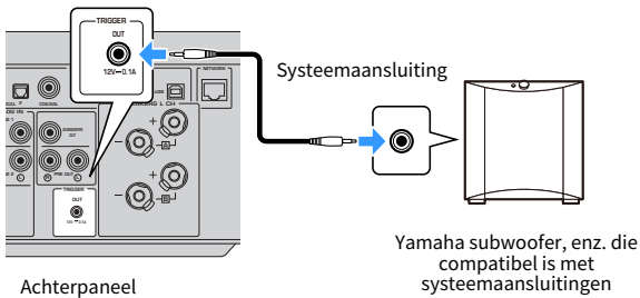
TRIGGER OUT-aansluitingen
