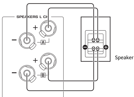
Achterpaneel
