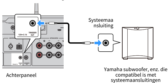
TRIGGER OUT-aansluitingen
