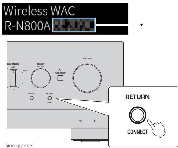
Voorpaneel
