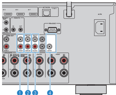
Het toestel (achterzijde)
